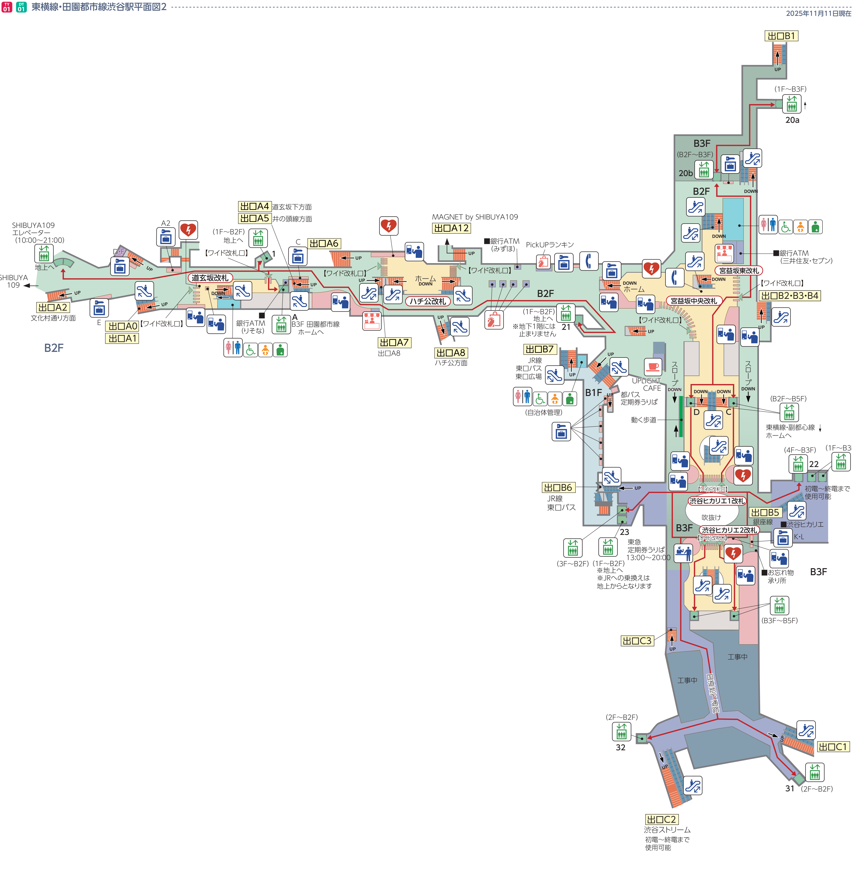
東横線・田園都市線渋谷駅平面図2 2025年11月11日現在
