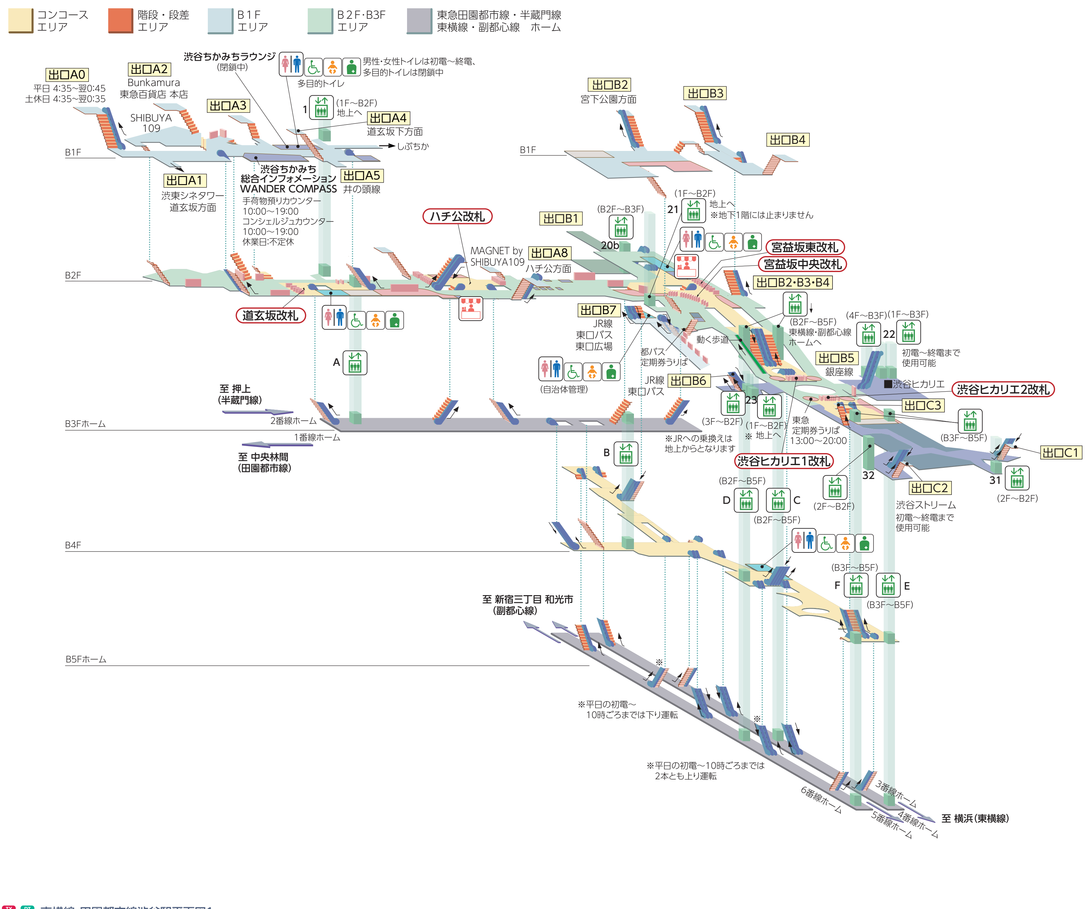
東横線・田園都市線渋谷駅平面図1 2025年11月11日現在
