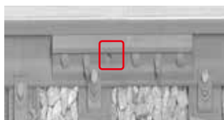
カメラ（静止画）によるボルトなどの抜けを検出
