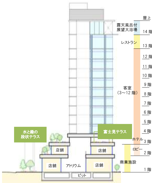
▲施設構成イメージ図
