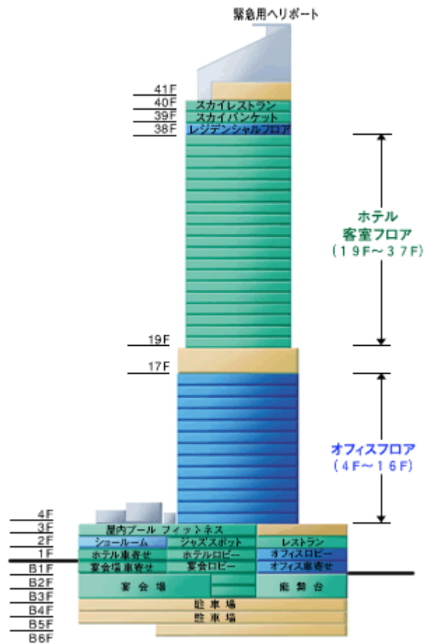
セルリアンタワーにおけるマルチキャリア環境のイメージ
